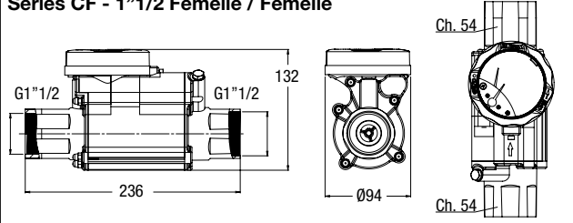
Séries CF - 1 1/2" Femelle / Femelle
