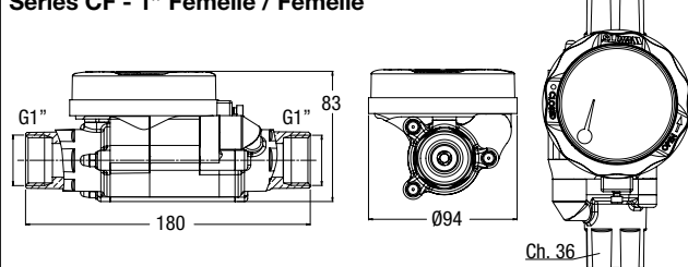
Séries CF - 1" Femelle / Femelle
