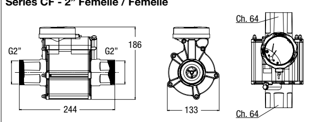
Séries CF - 2" Femelle / Femelle
